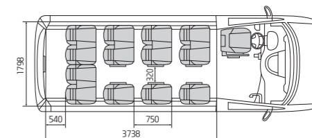
Uspořádání s předními dveřmi
