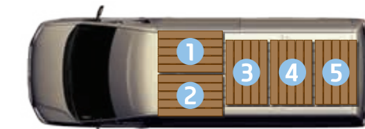
Dlouhý rozvor (5 europalet)
