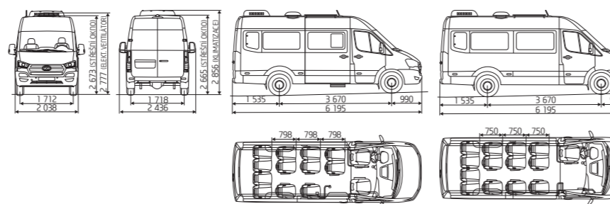
Verze s dveřmi vpředu a bočními posuvnými dveřmi
